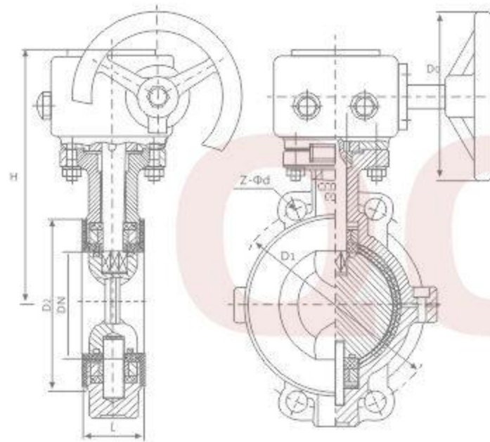
DA371 F4 F/P 型对夹式蜗轮传动蝶阀 (中线)
